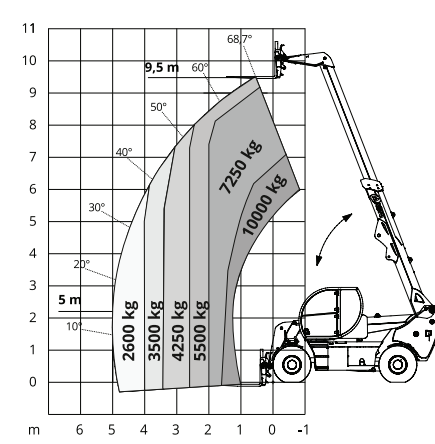
Telehandler MAGNI 10.10
