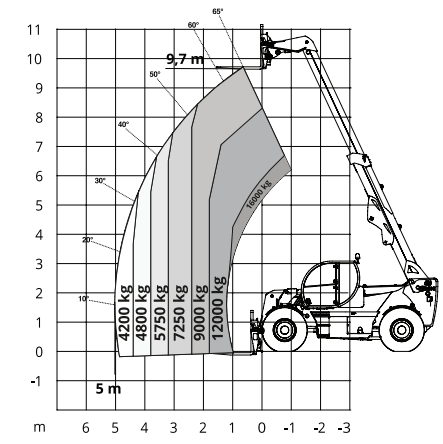
Telehandler MAGNI 16.10
