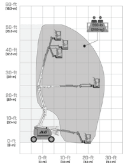
Articulating Boom Lift JLG E450AJ
